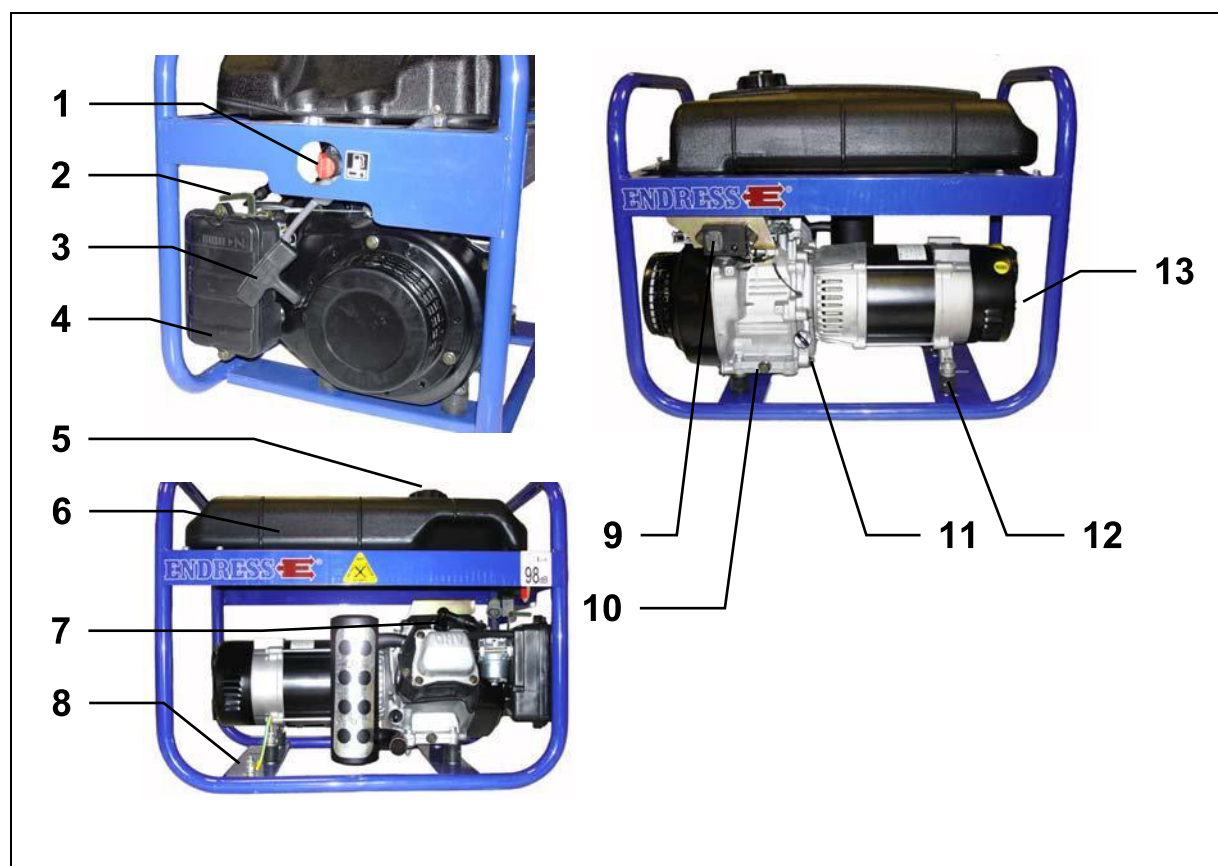
Abb. 3.1: Bestandteile des Stromerzeugers
