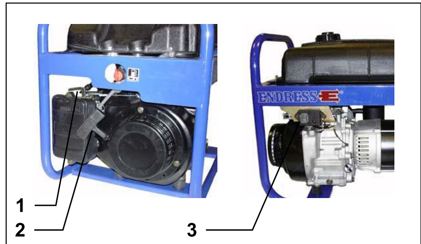
Abb. 4.2: Motor starten
