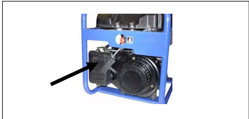
Abb. 4.8: Luftfilter entfernen
