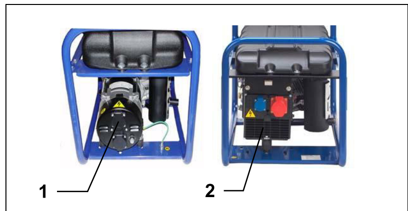
Abb. 4.3: Verbraucher anschließen
